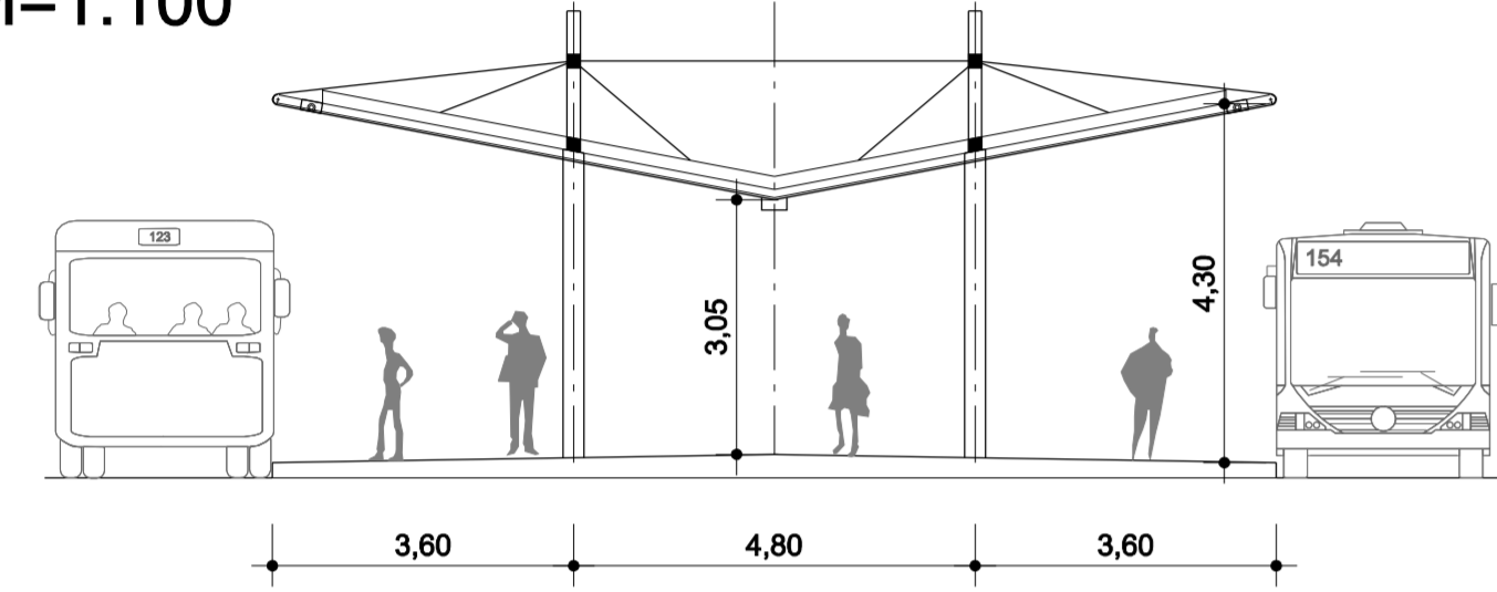
Überdachung Q1 M=1:100
